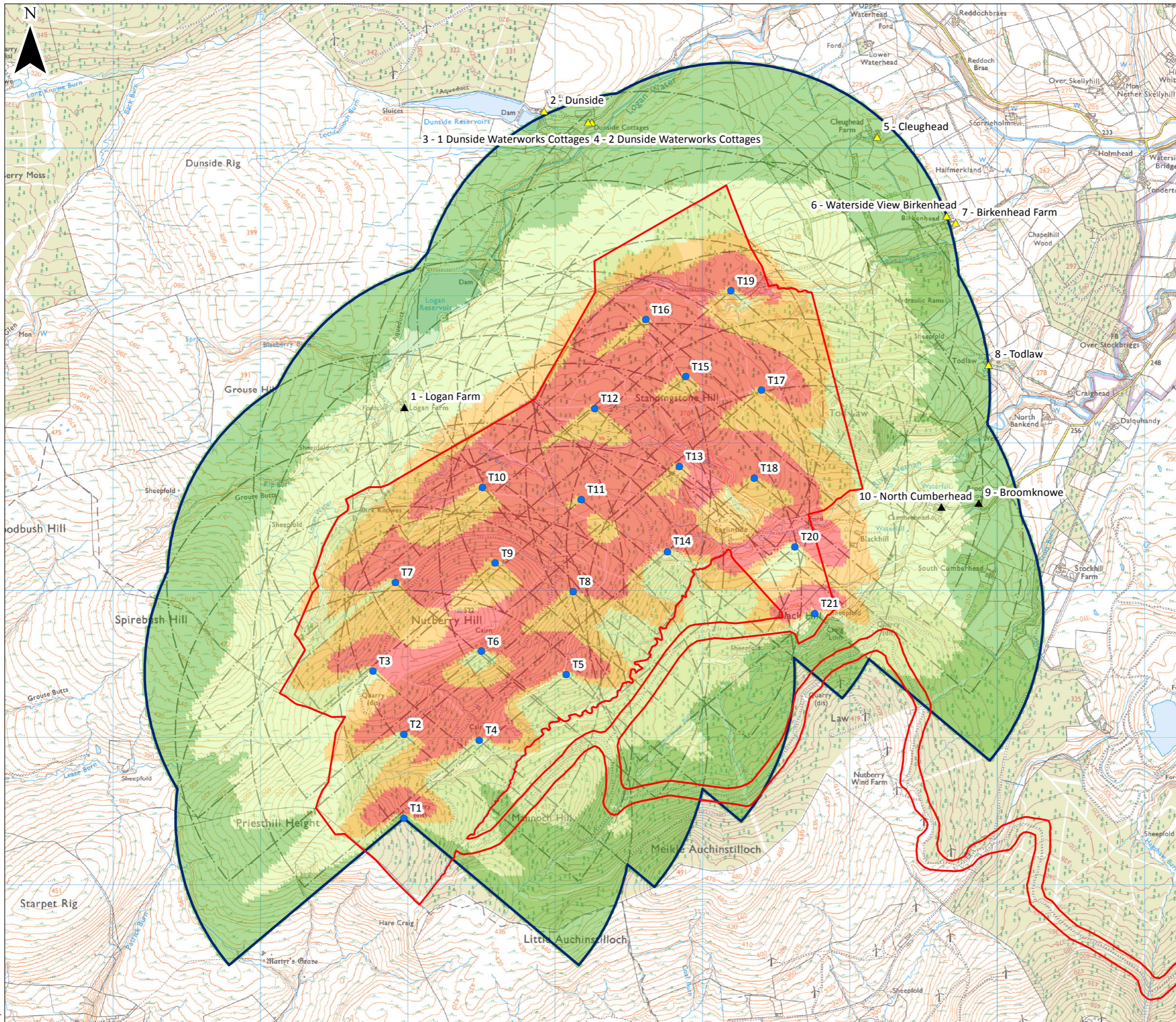
Shadow Flicker Map (Realistic Scenario)
